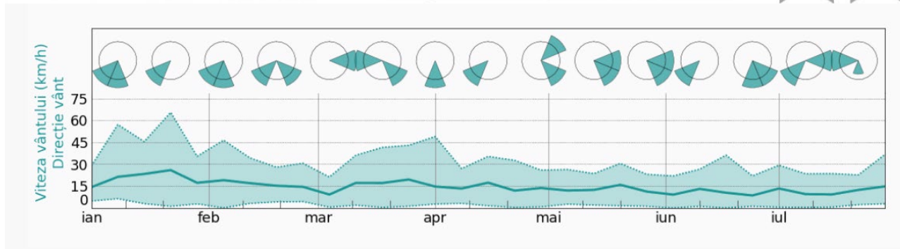
Figura 37 - Viteza și direcția vântului anul 2024 Ciurea
