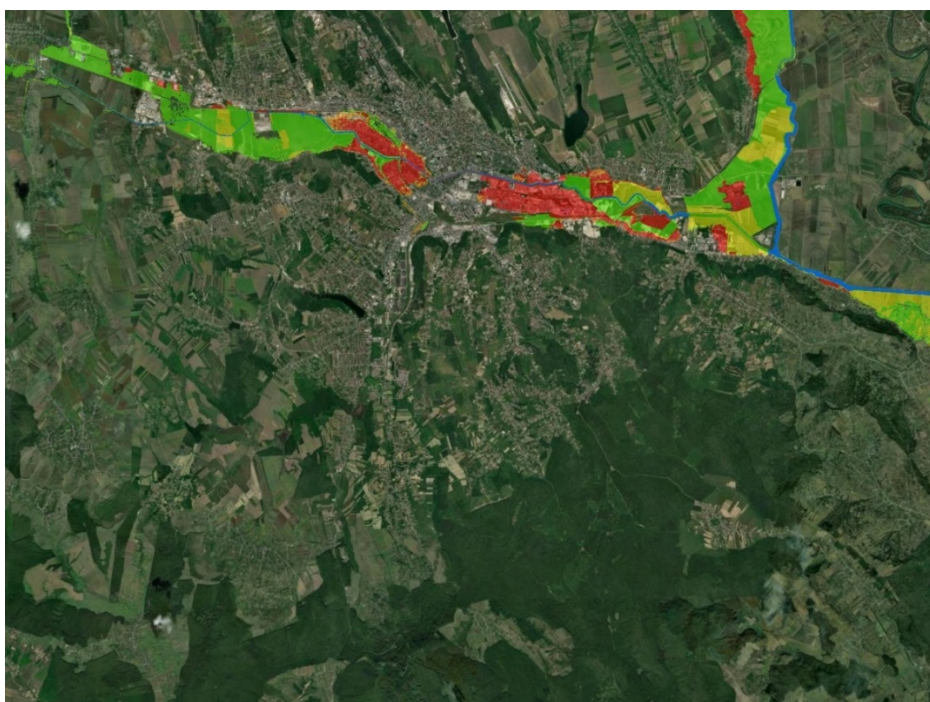
Figura 26 – Zona inundabilă și riscul asociat cu un grad de asigurare de 0,1%
