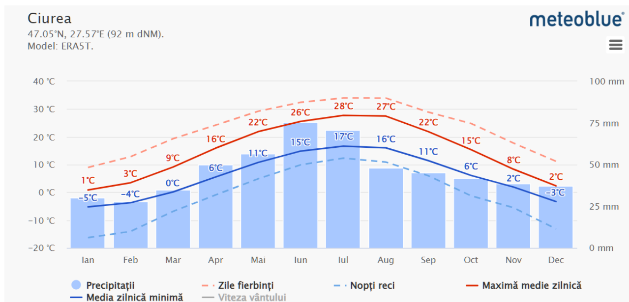
Figura 36 - Graficul precipitațiilor lunare pentru comuna Ciurea (2011 – 2021)
