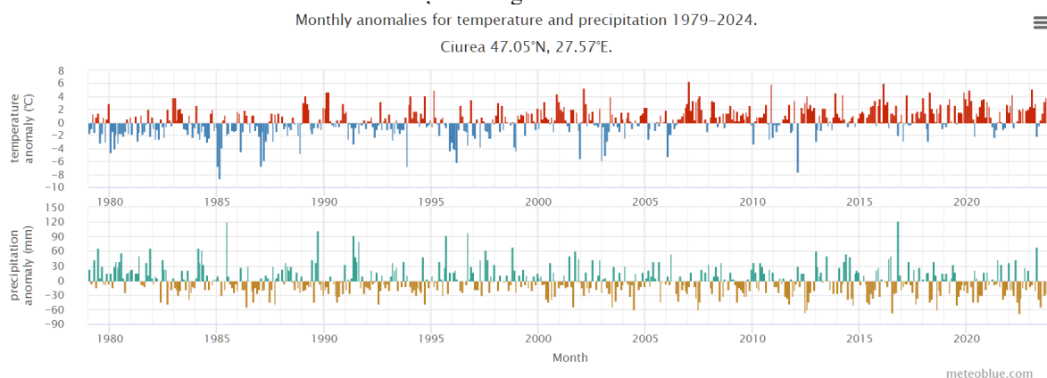
Figura 31 - Anomalii lunare de temperatură și precipitații - Schimbări climatice Ciurea
