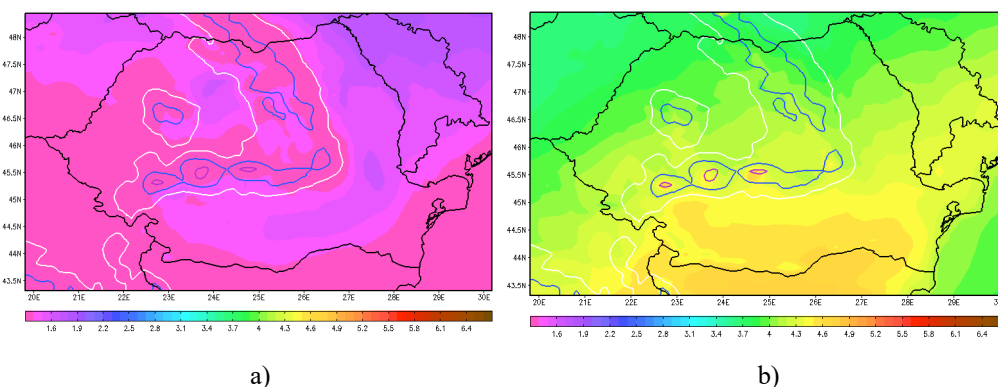
Figura 33 - Creșterea medie a temperaturii aerului a) iarna, în intervalul 2021-2050 față de intervalul 1971-2000 și b) vara, în intervalul 2070-2099 față de intervalul 1971-2000
