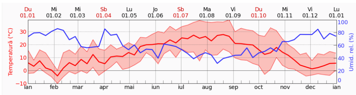
Figura 34- Umiditatea relativă în anul 2023 – Ciurea
