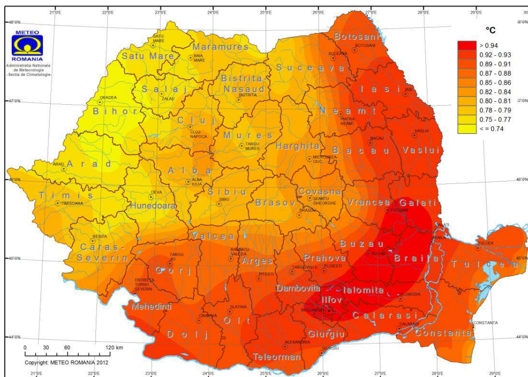
Figura 32 - Creșterea temperaturii medii multianuale (°C) în intervalul 2001-2030, comparativ cu intervalul de referință 1961-1990 Sursa: https://www.meteoromania.ro/despre-noi/cercetare/climatologie/
