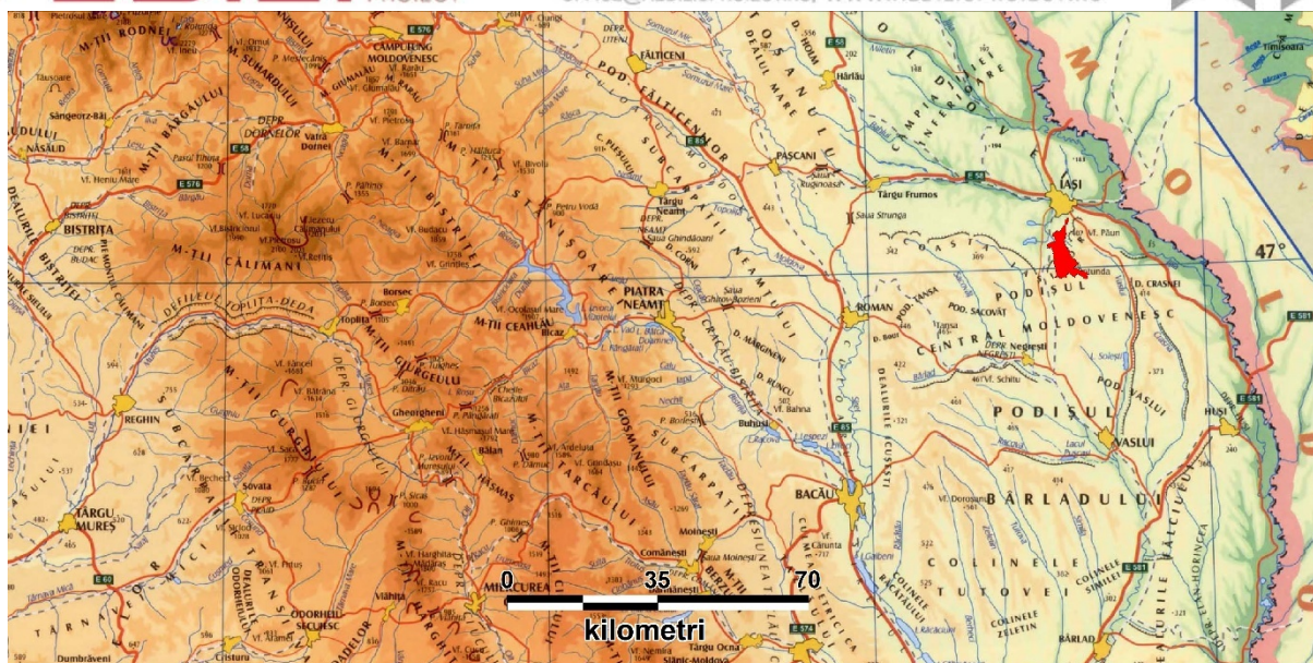
Figura 1 – Amplasarea zonei studiate în cadrul unităților majore de relief Sursă: Harta fizică a României – Prof. Univ. Dr. Mihai Ielenicz
