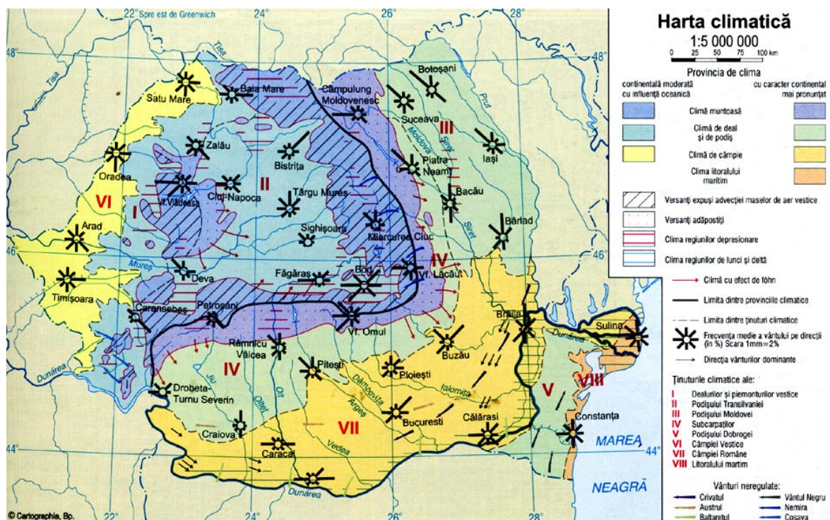
Figura 3— Harta climatică a României
