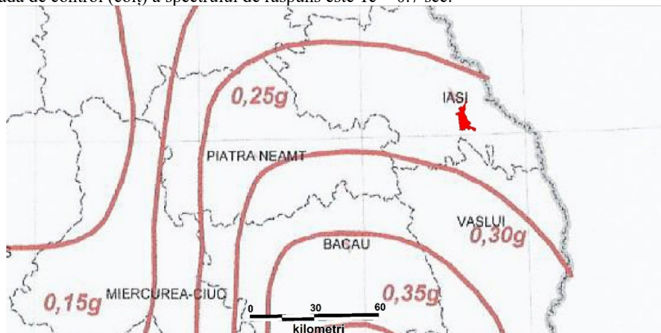
Figura 24 – Cod de protecție seismică – valoare de vârf a accelerației terenului
